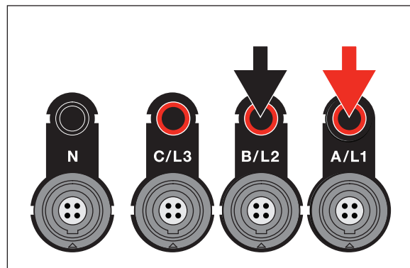
图示 7. 不带中性点电压的线路电源
