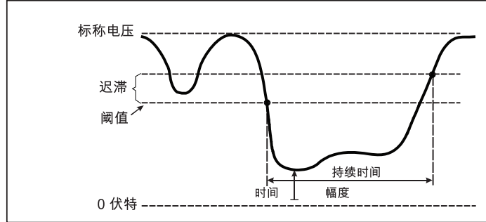
图示 11. 电压中断的特征
