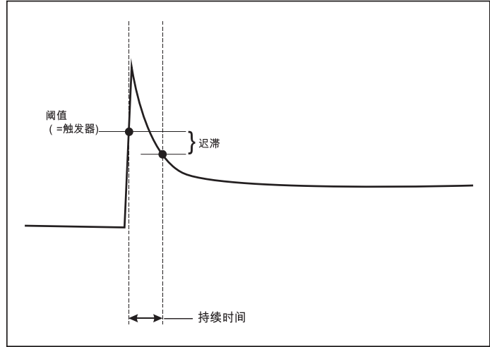
图示 14. 浪涌电流特性
